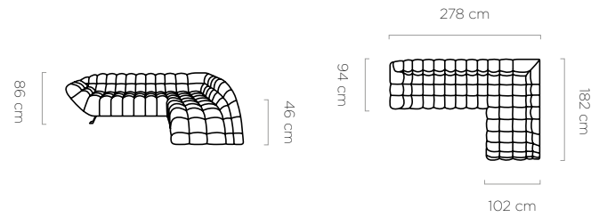
noga / leg / fuß: 12 cm
