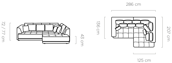
powierzchnia spania / sleeping area / schlaffläche: 124 X 217 cm
