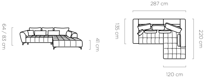
powierzchnia spania / sleeping area / schlaffläche: 126 X 228 cm
